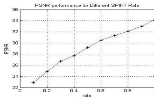
Fig 8: PSNR v/s rate(r)
